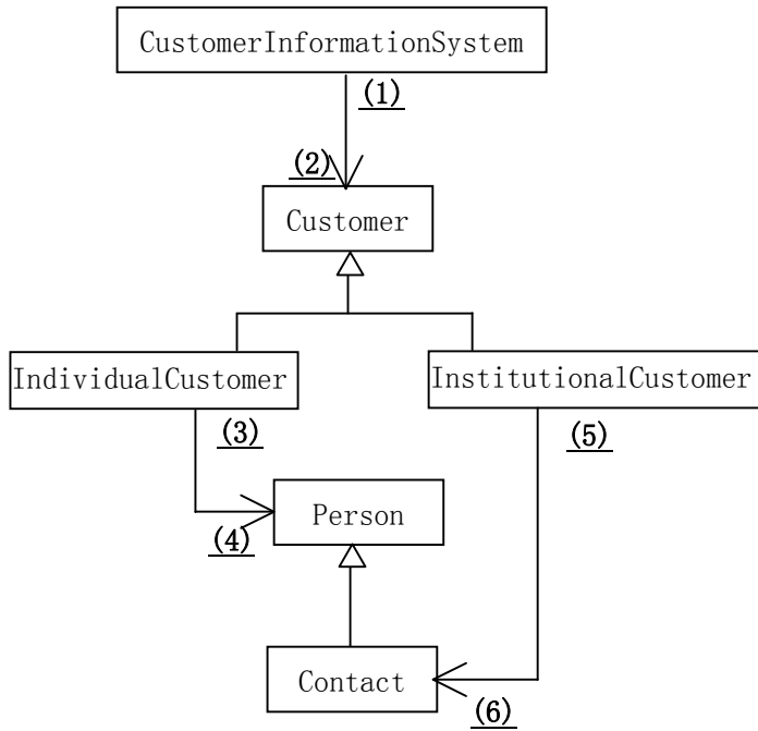
图 2-1 客户信息管理系统的 UML 类图
