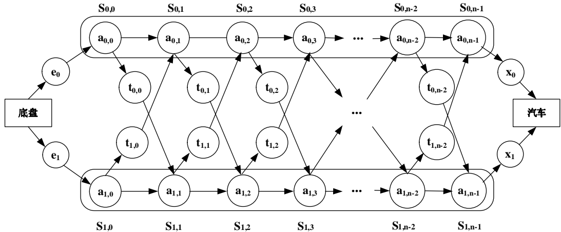
图 4-1 汽车装配线
