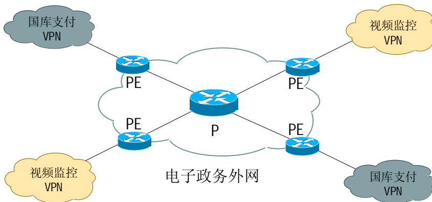
图1-1 电子政务外网承载VPN示意图
